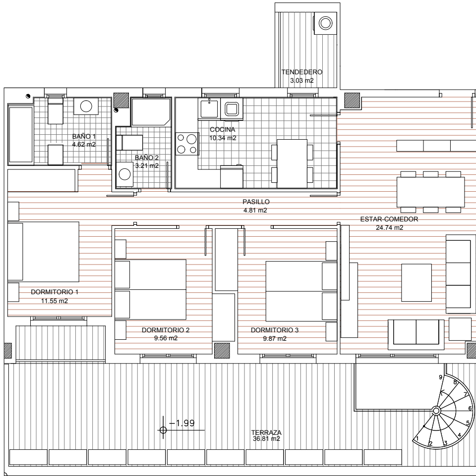
Planta de vivienda
