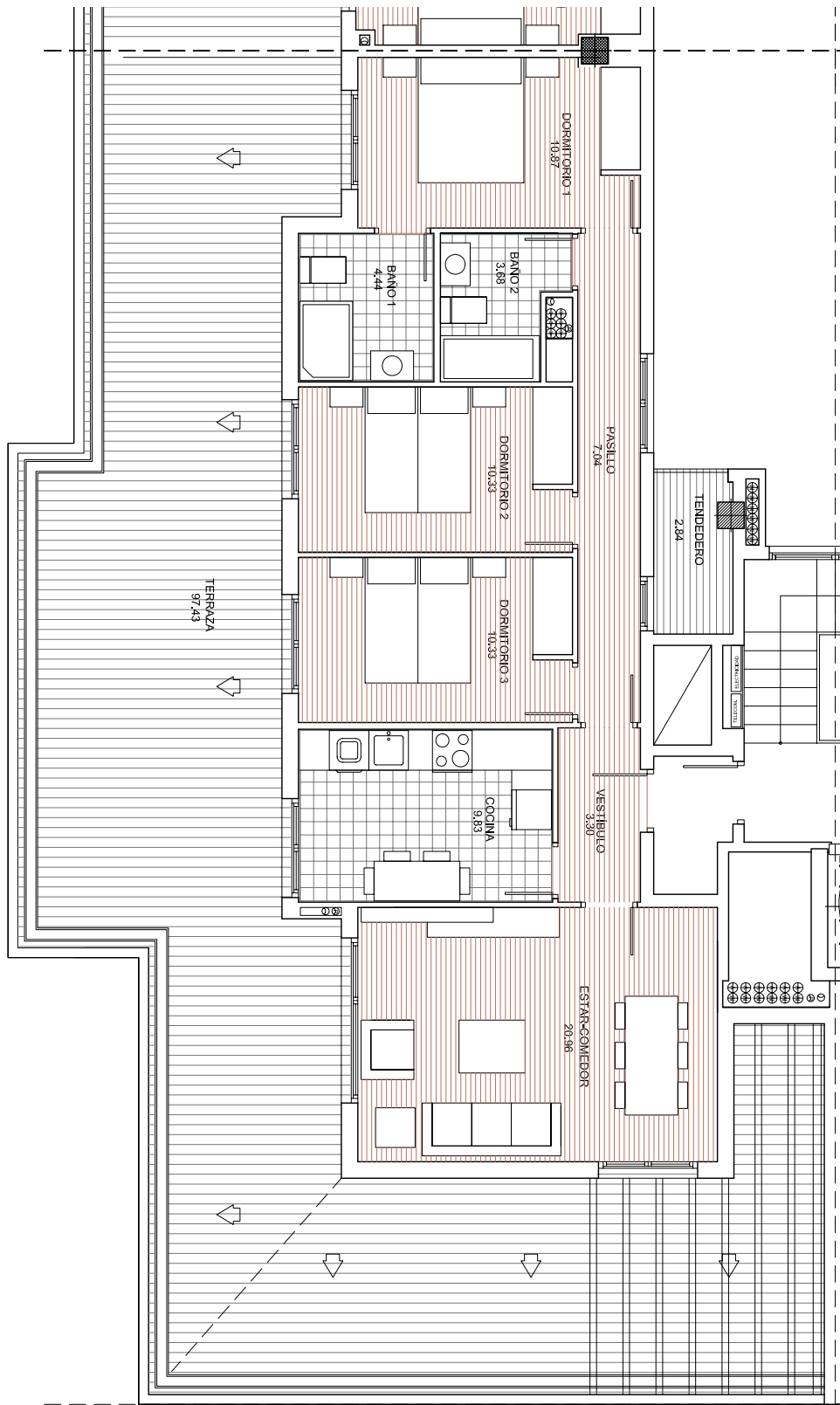
Planta de vivienda
